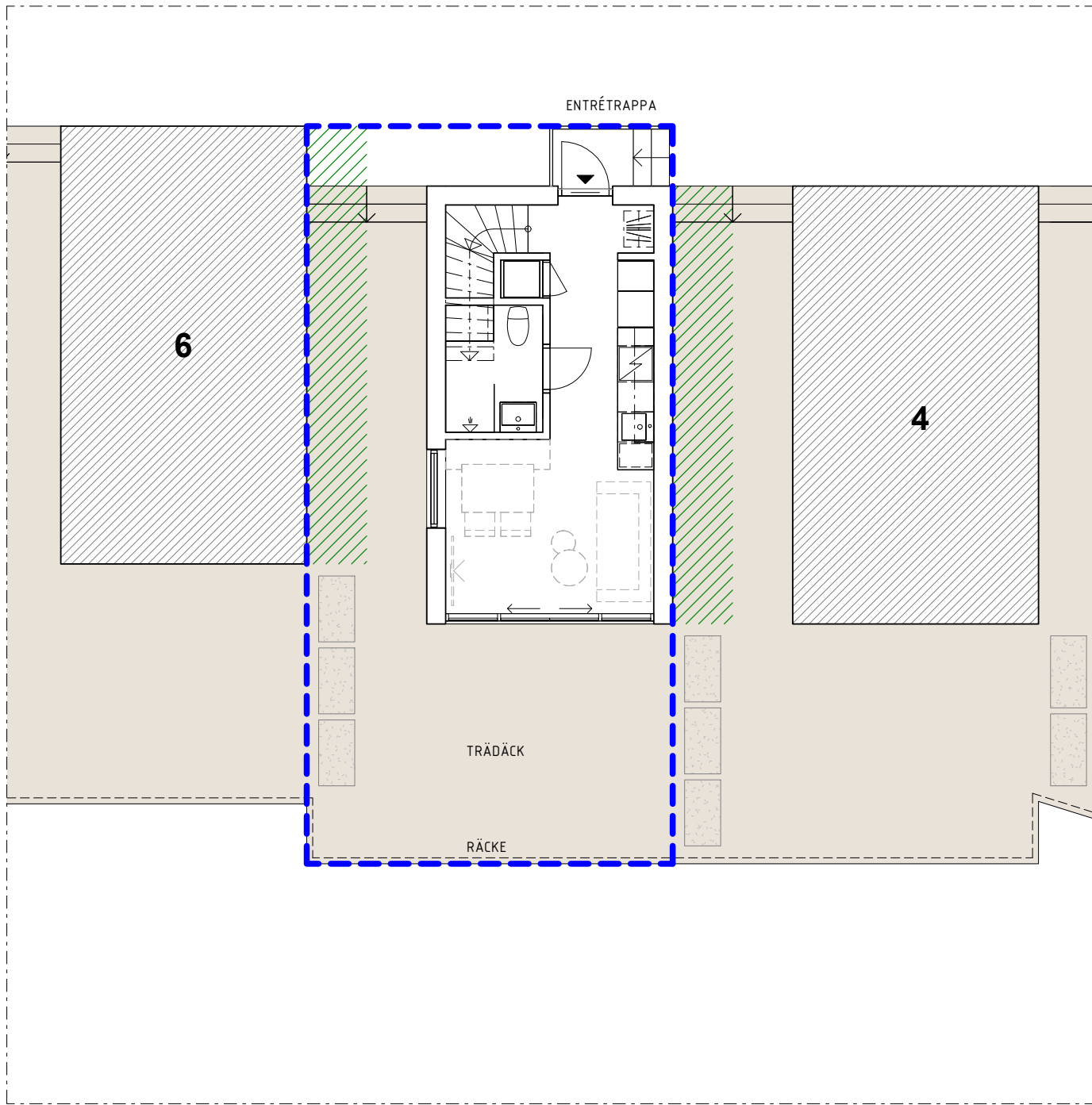
PLANRITNING FISKESTUGA 5
