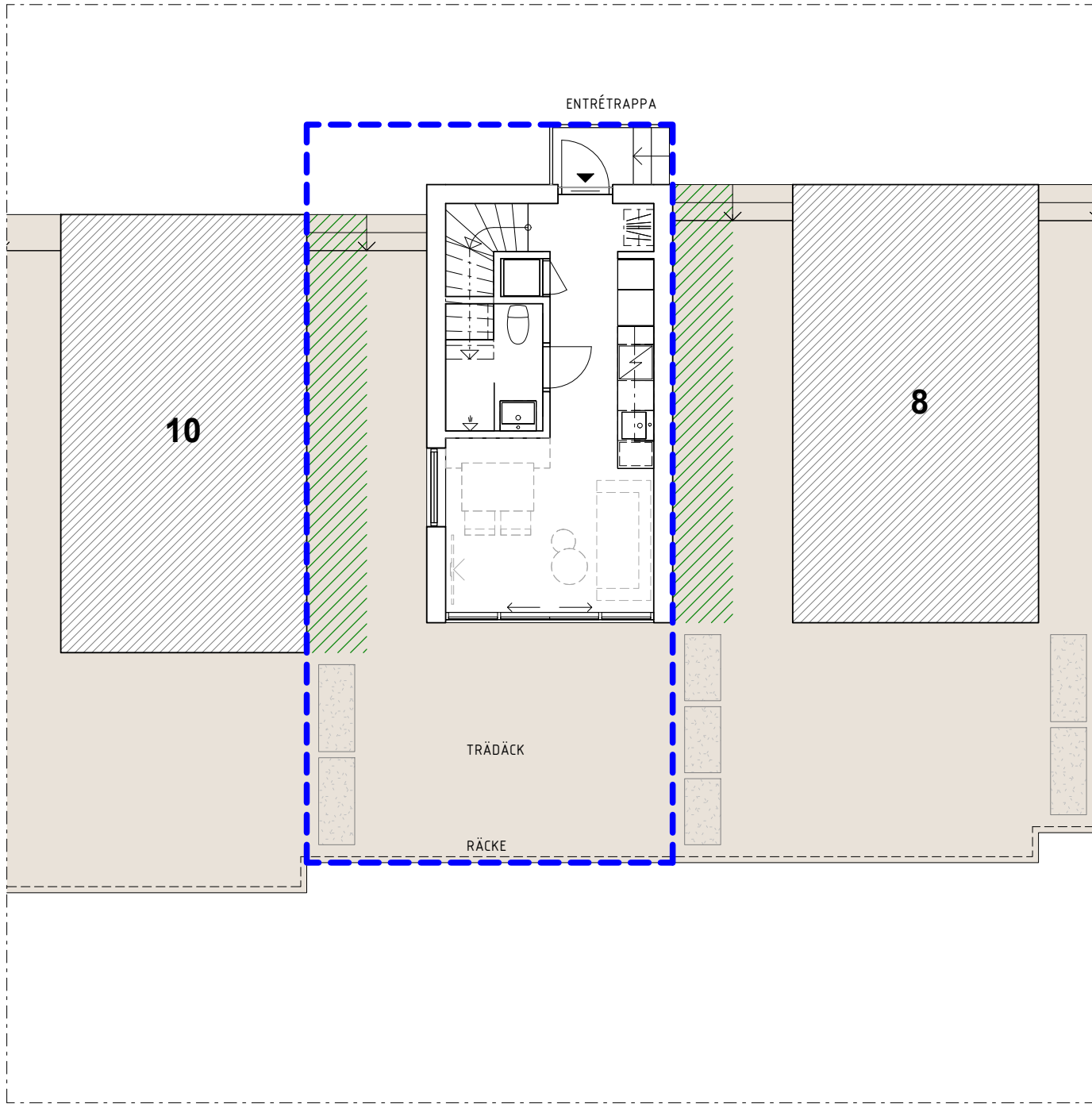
PLANRITNING FISKESTUGA 9
