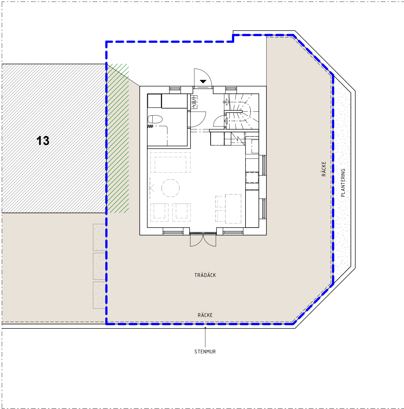
PLANRITNING HAVSHUS 12
