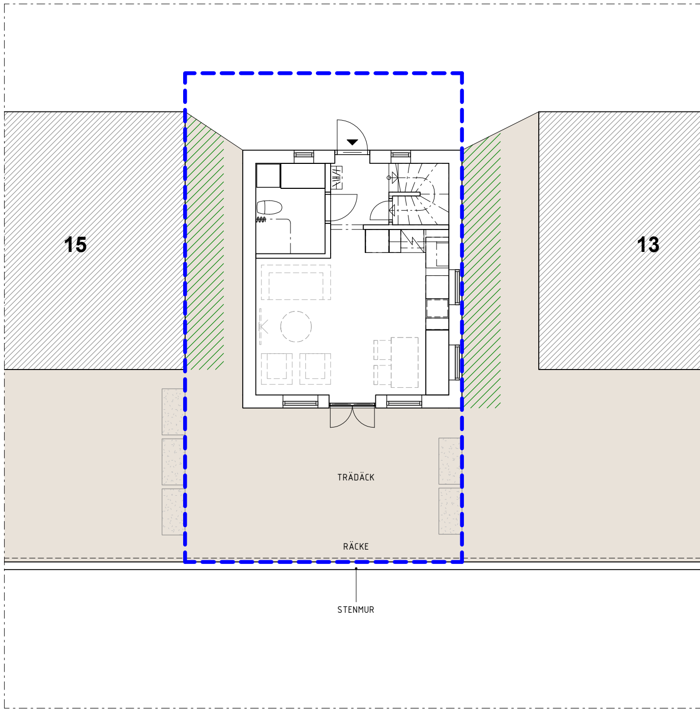
PLANRITNING HAVSHUS 14
