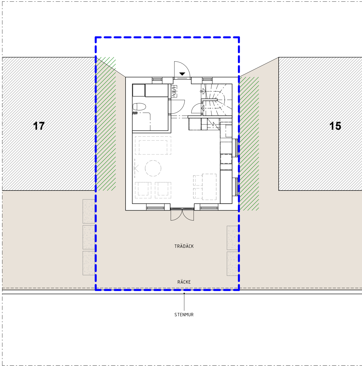
PLANRITNING HAVSHUS 16
