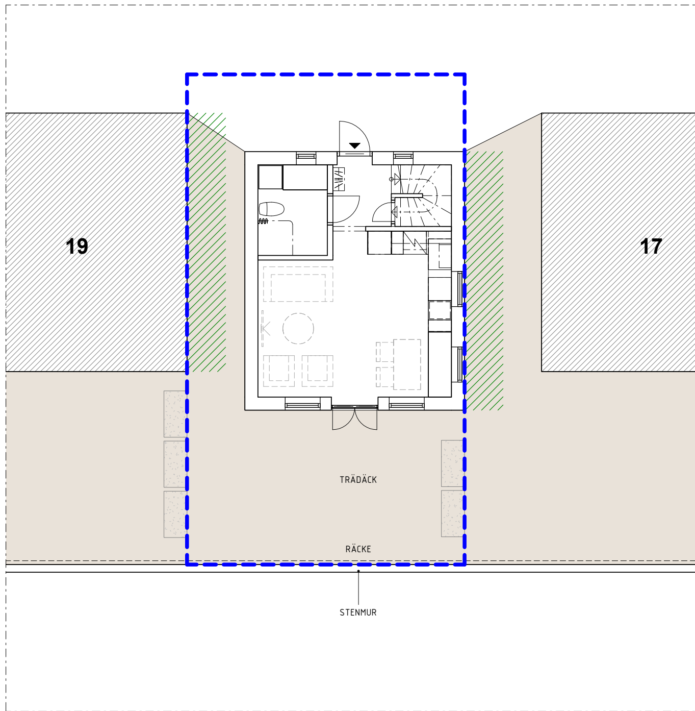
PLANRITNING HAVSHUS 18
