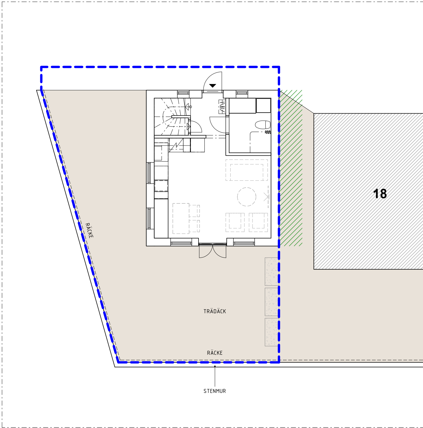
PLANRITNING HAVSHUS 19
