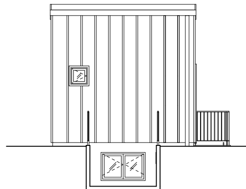
FASAD NORR
