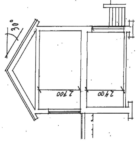
SEKTION KALA 1:100
