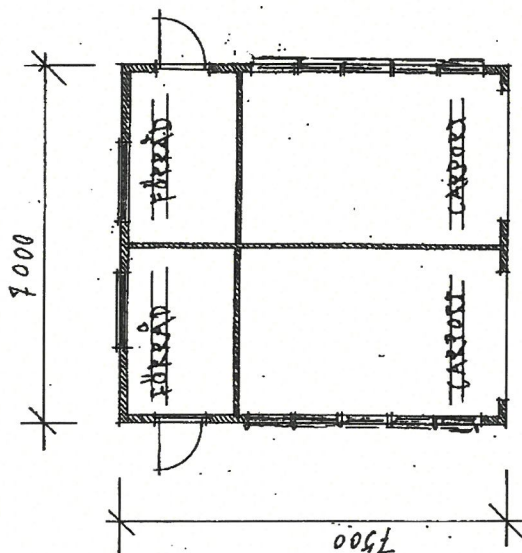
PLAN SKALA 1:100
