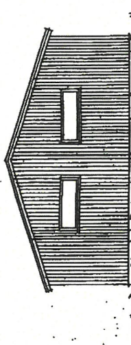
SÖDVÄSTFASAD SKALA 1:100
