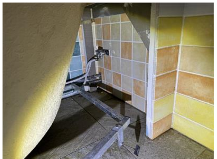
Rör genomföringar i vägg vid badkaret i badrum.
