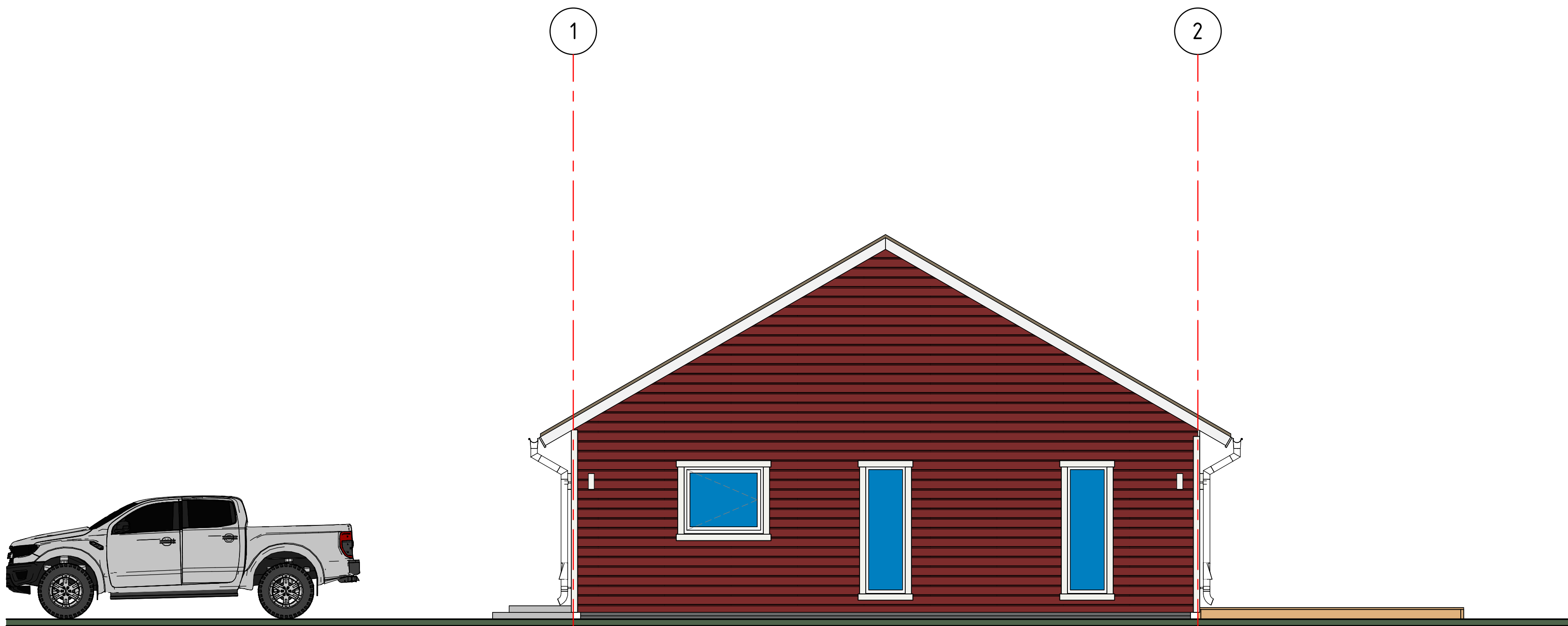
Fasad vy 4 1 : 50
