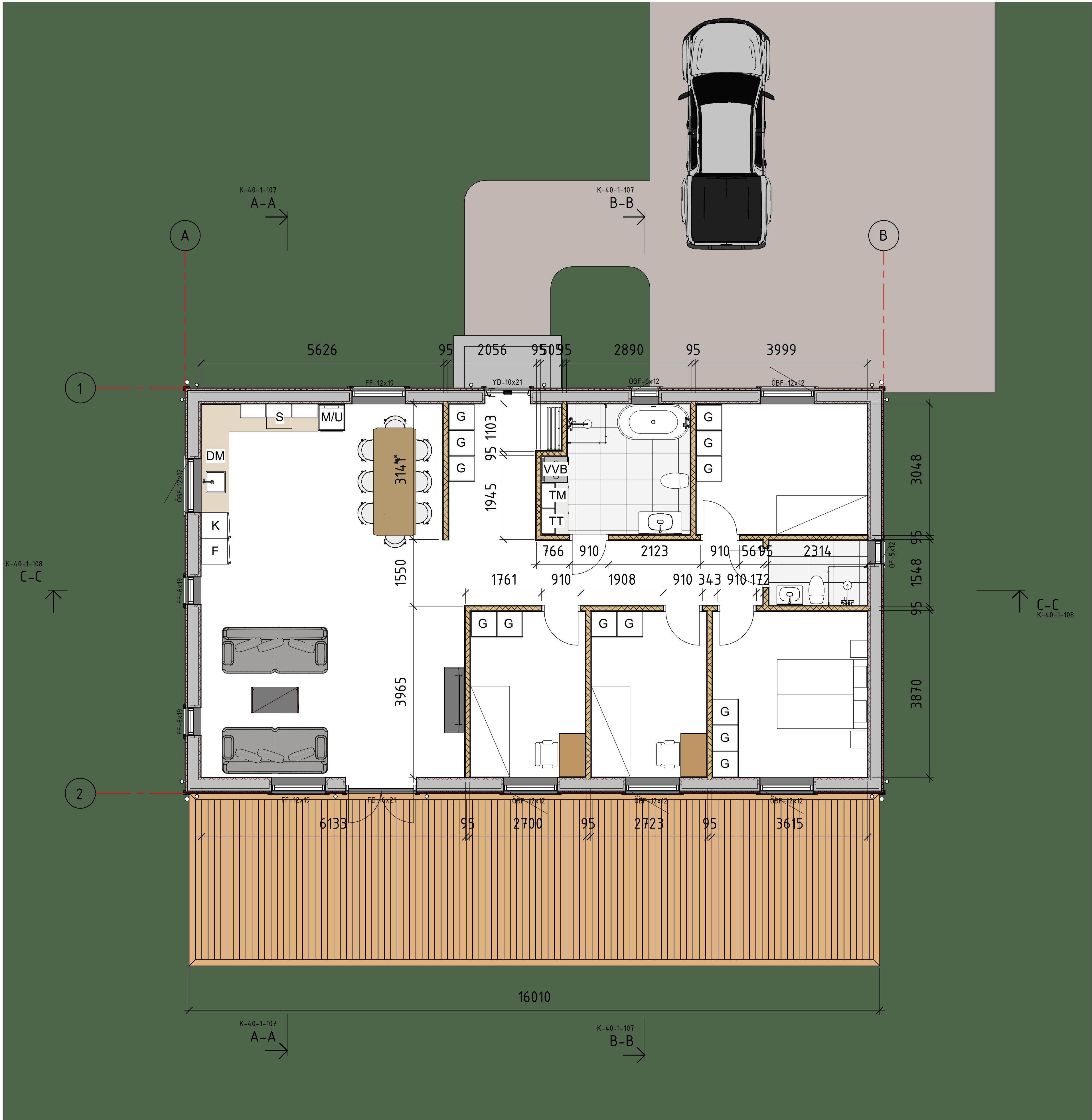
Plan 1 Måttsättning 1 : 50
