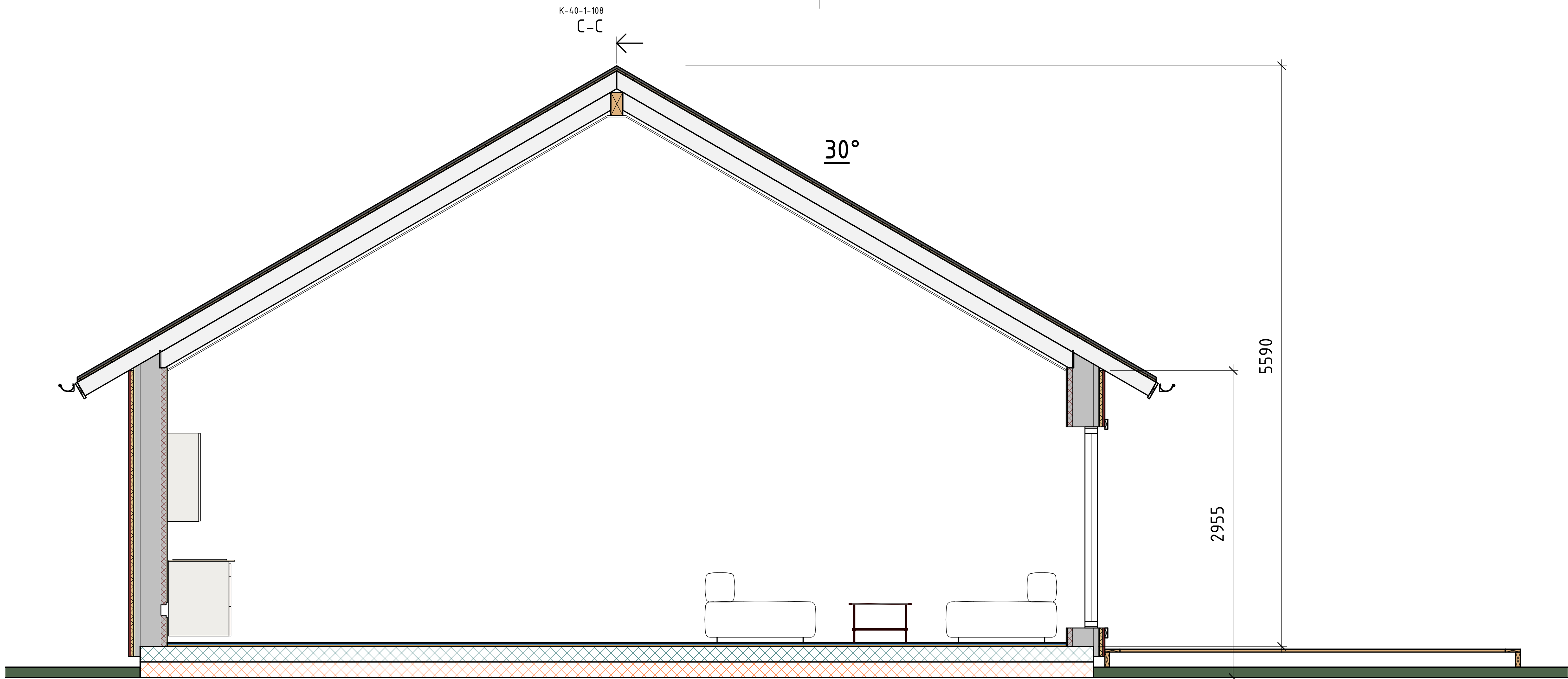
A-A 1 : 25
