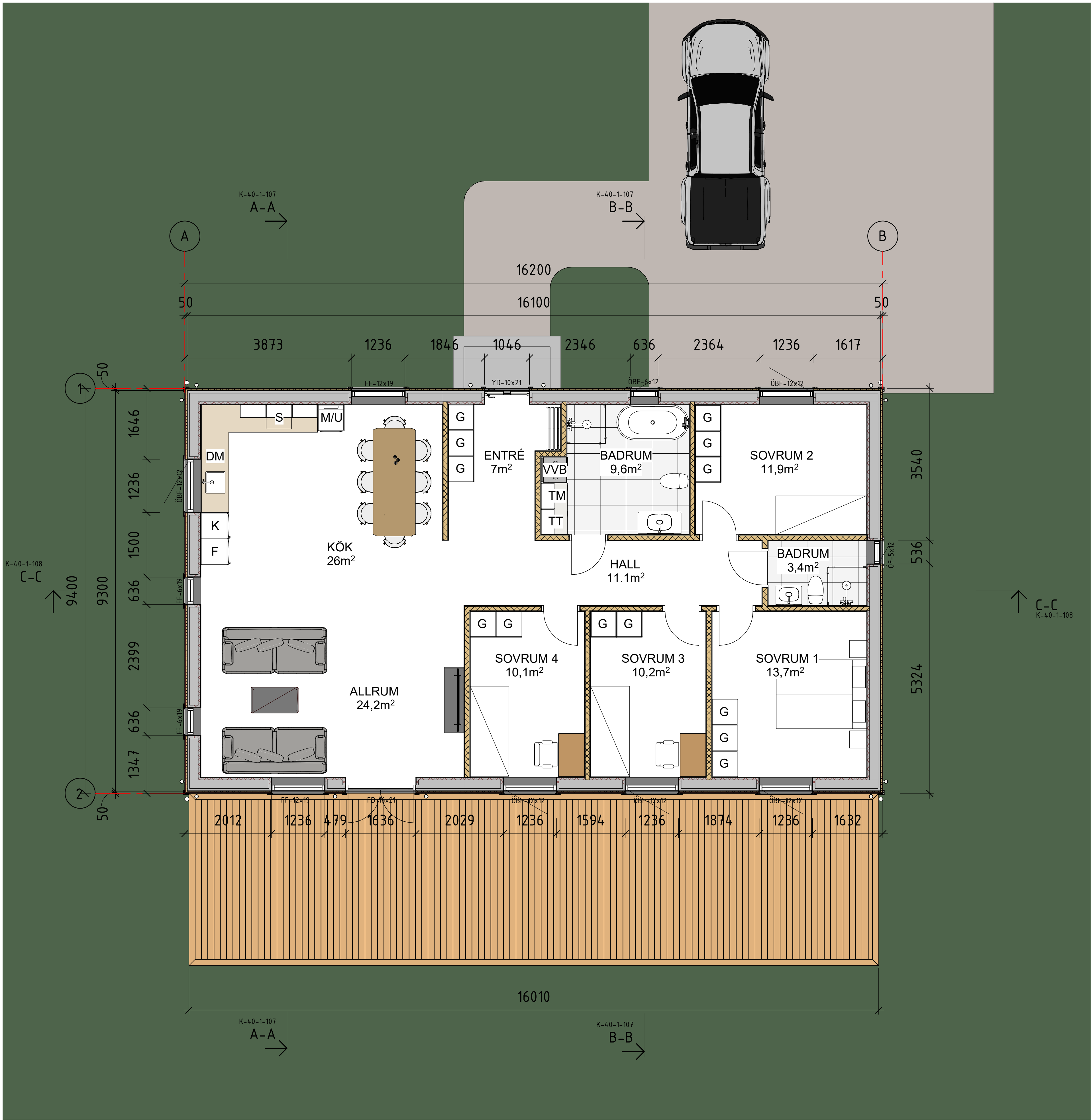
Plan 1 1 : 50
