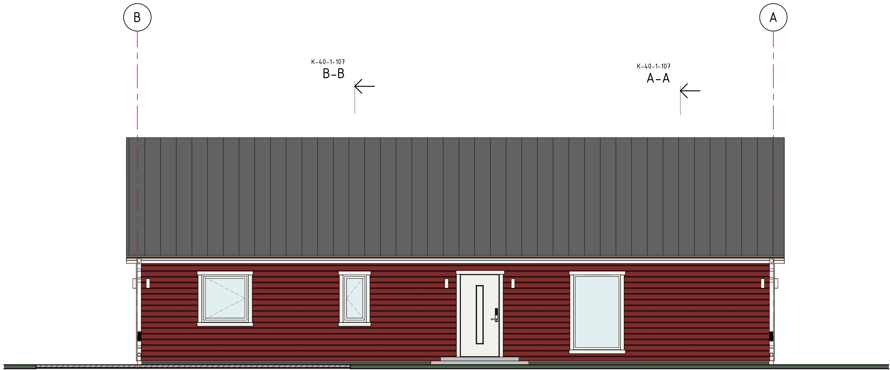
Fasad Vy 1 1 : 50
