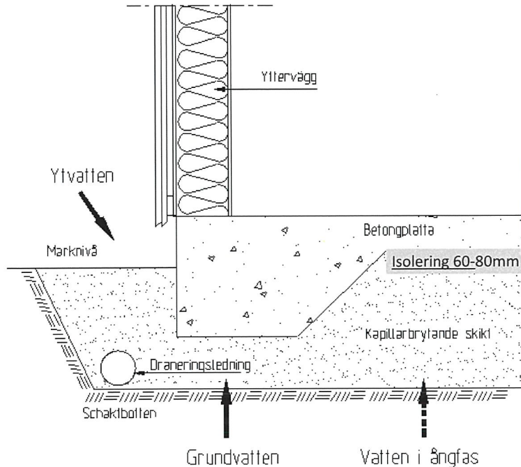
Figur, Fuktblastningar mot en platta på mark
