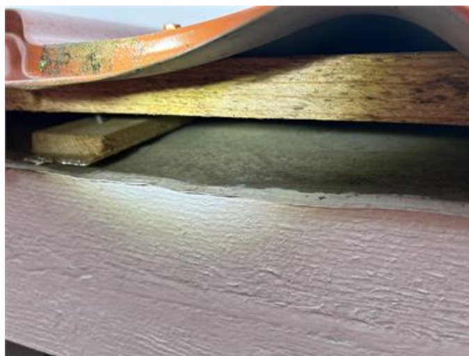
Tak: Under korrigerad plåt ser man armerad plast på underlagstaket.
