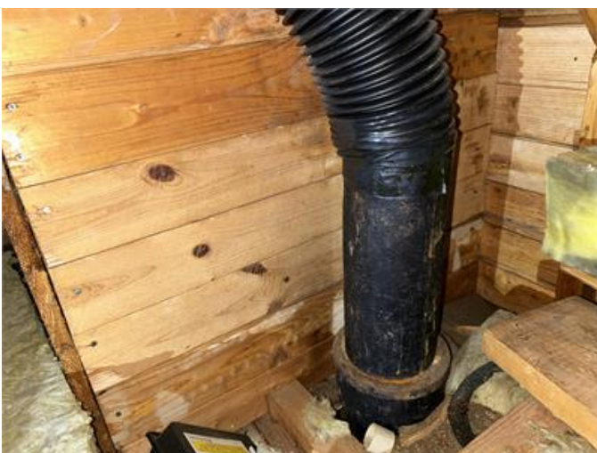
Nockvind: Gjutjärnsrör till avloppsluftare.
