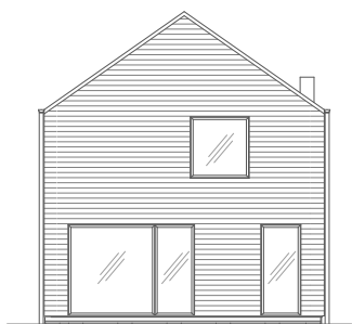
FASAD TRÄDGÅRDSSIDA
