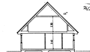
SEKTION
