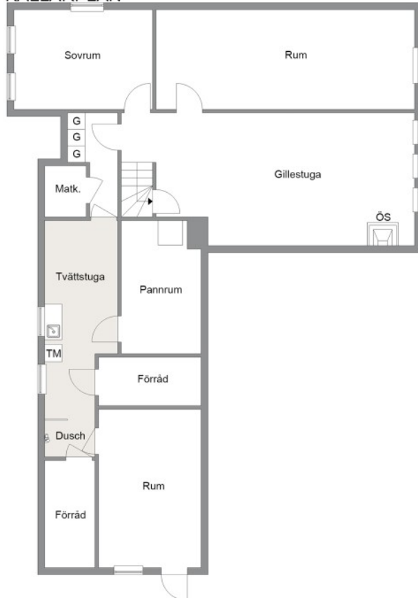
KÄLLARPLAN
