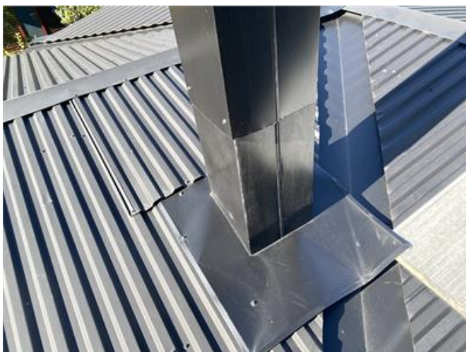
Anslutning skorsten/ tak
