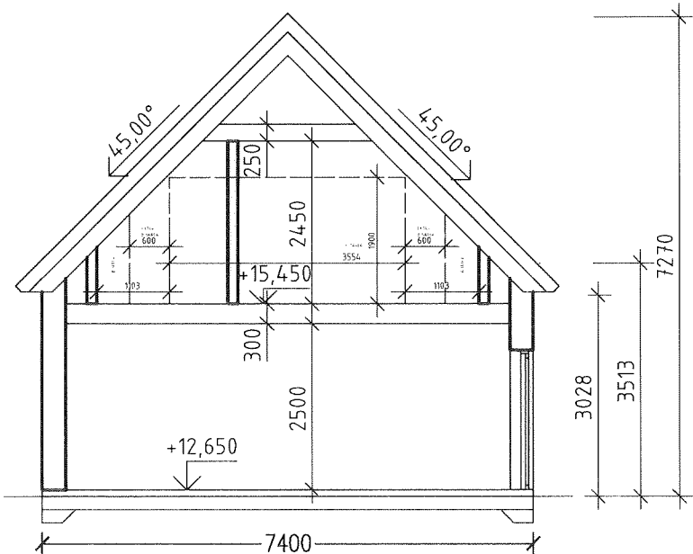
SEKTION A-A
