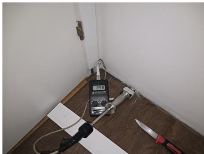
Fuktmätning i innerväggssyll.
