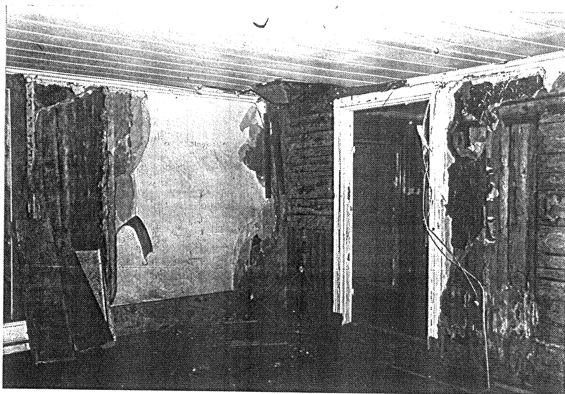
Samma rum mot SÖ, svåra rötskador i vägg mot förstugan. Obs det gamla, lägre dörrläget mot förstugan till höger om det nuvarande!
