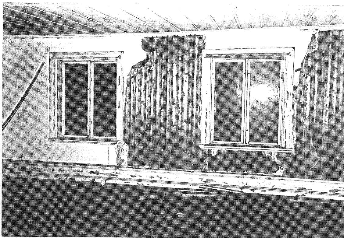
Gamla ytskikt i salen (207). Spontat furugolv, treetex i taket, omålad pärlspontpanel under många tapetskikt på pappmakulatur.
