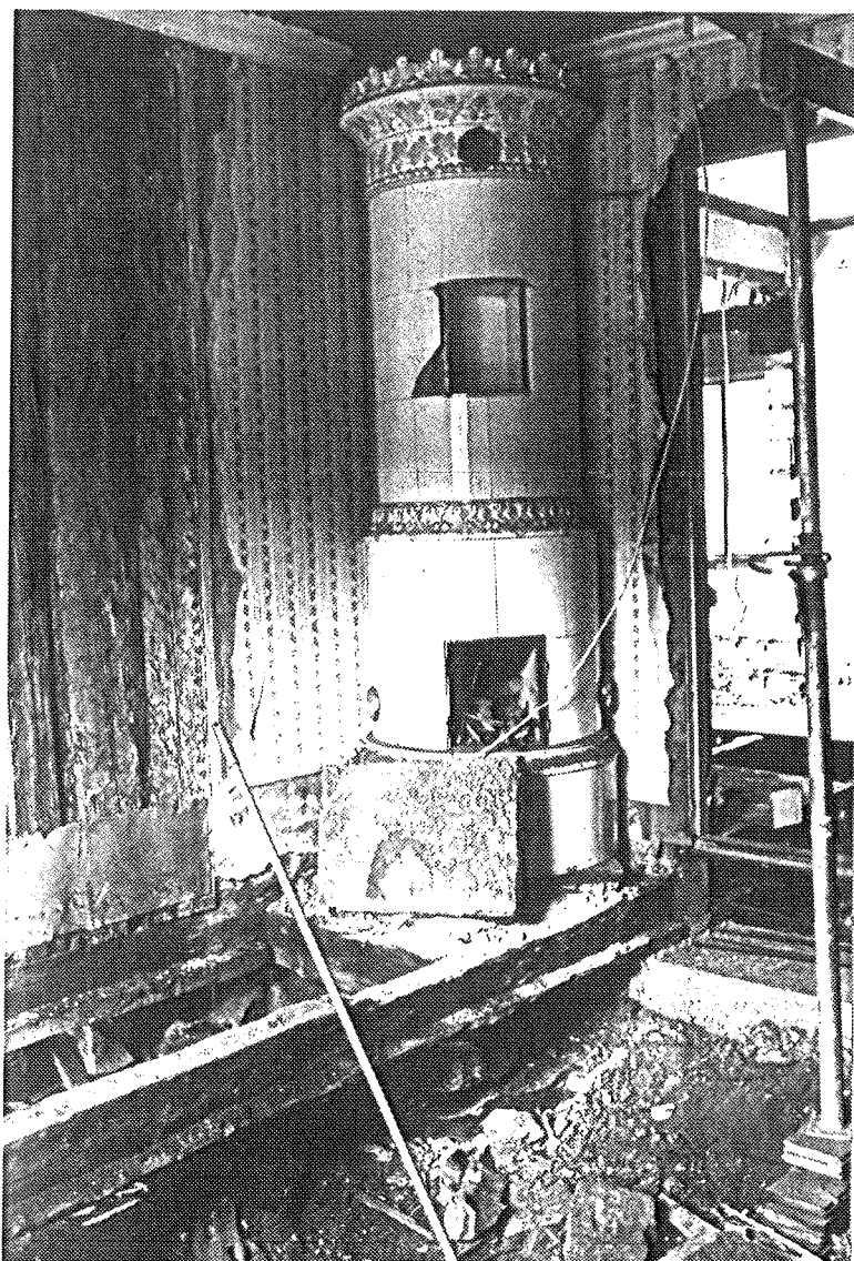
Rum 206, äldre bjälklag med avväxling för kakelugnen. Ny betonggjuten sockel under mellanvägg till höger.
