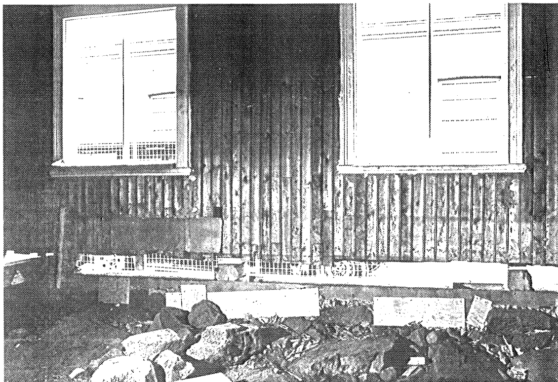
Salen (207) sedan syllstocken demonterats och stensockeln avjämnats med betongpågjutning. Obs den gamla isoleringen av ytterväggen, i form av omålad pärlspontpanel.
