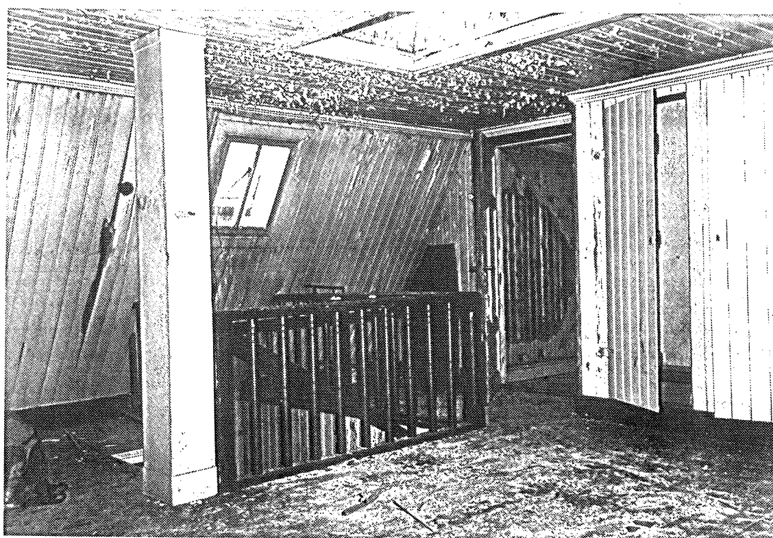
Vindsvåningens stora öppna hall med pärlspont å väggar & tak. Fönster i takfallet och sekundär avloppsluftningskanal vid trappan.
