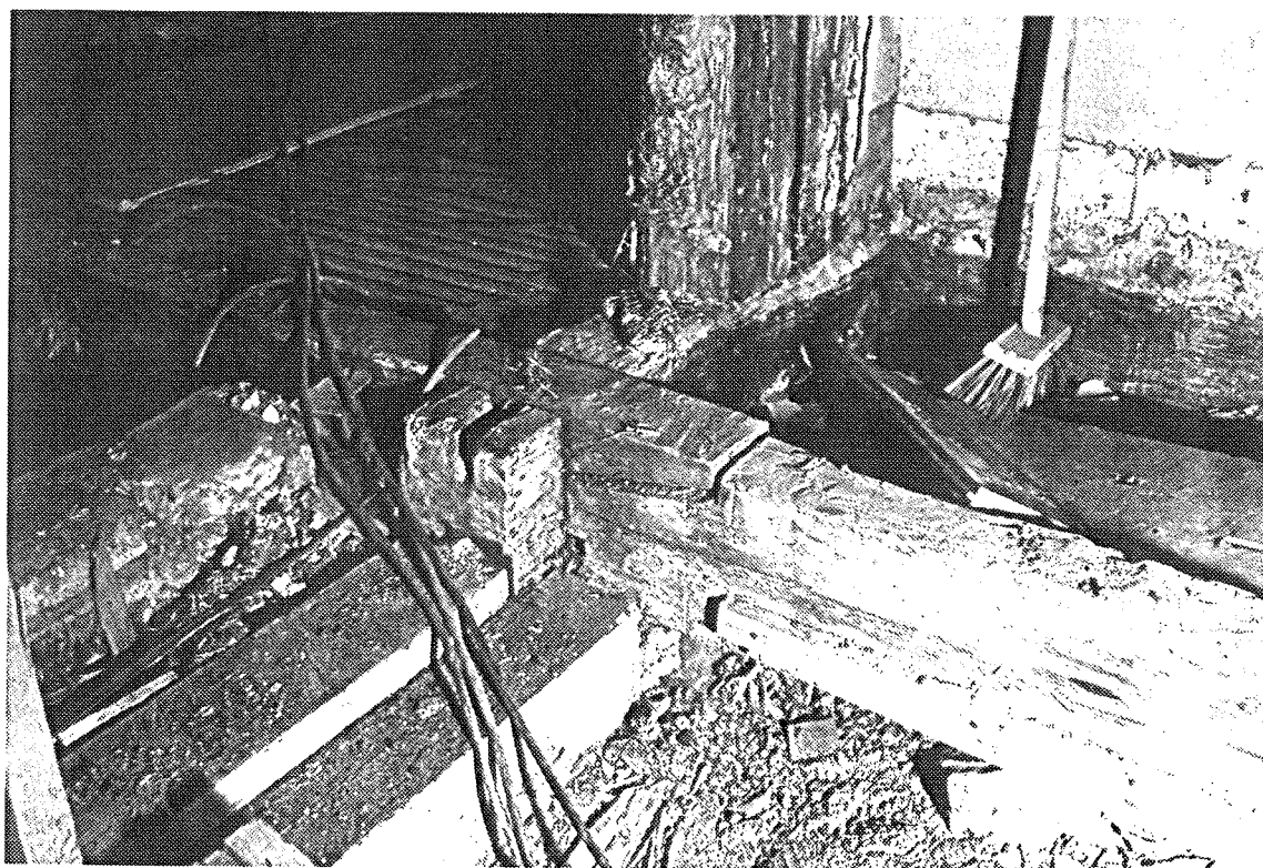
Äldre bjälklag skarvat över mellanvägg (mellan serverings- gång och sal). Blixtskarv!
