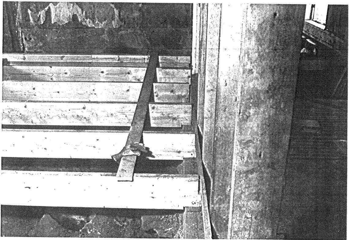
Nytt bjälklag i salen, sett mot den rivna, uppstämpade väggen mot förstugan. De nya bjälkarna mäter 45x220 och ligger på ett cc-avstånd om 600mm. Nedan Bjälkarnas upplag på ny grundmur av betong under mellanväggen.
