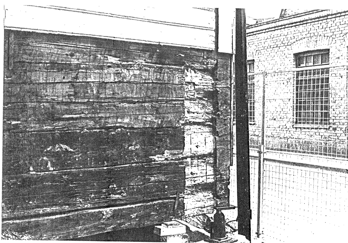
Hörn som ovan, hörnet lyft, gamla syllstocken borttagen. Laxad knutkedja.
