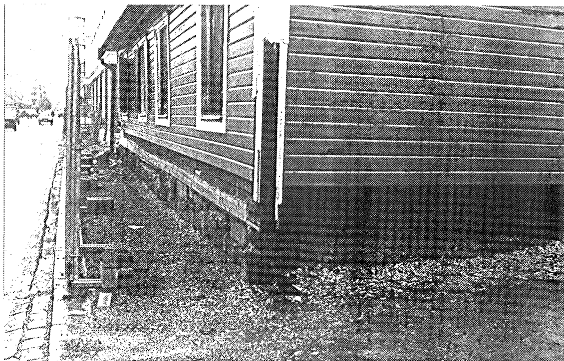
Samma fasad som ovan, med ny syllstock av sammansatt virke monterad.
