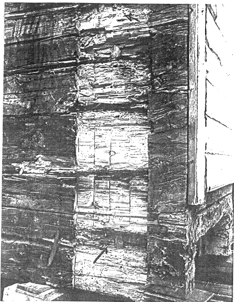
Detalj av NÖ hörnet, gavel- sidan. Rötad ytved bort- huggen och de sammanhållande dymlingarna frilagda!
