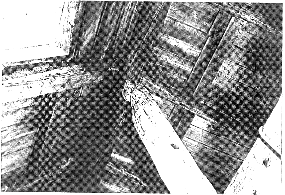
En av mittåsens stöttor, sedd underifrån.
