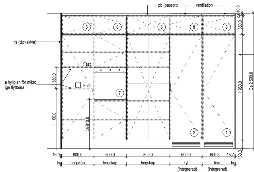
A-A ELEVATION
