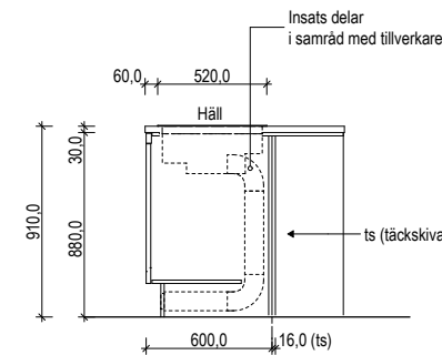
E-E SEKTION GENOM KÖKSÖ
