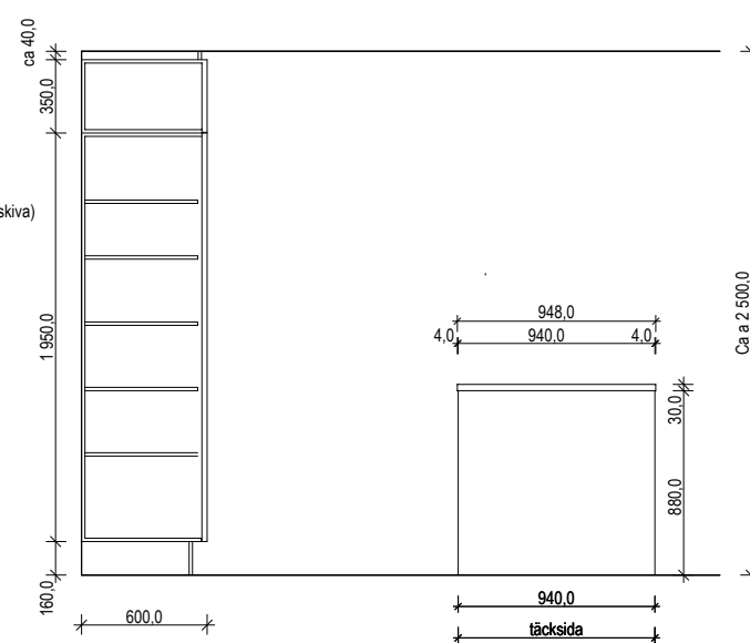
B-B ELEVATION-SEKTION
