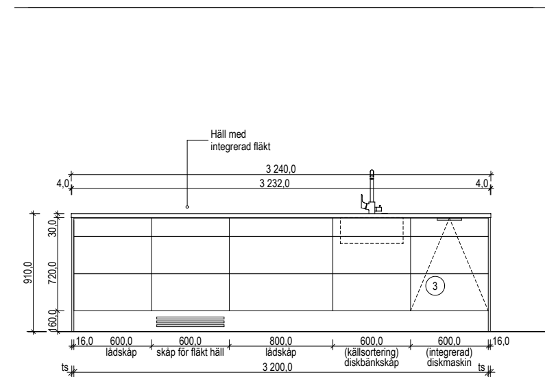
C-C ELEVATION KÖKSÖ MOT KÖK
