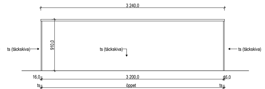
D-D ELEVATION KÖKSÖ
