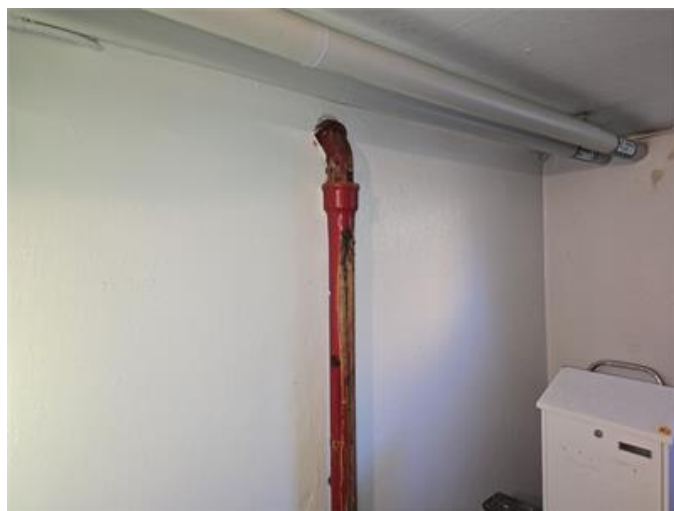
Exempel på rostangrepp i gjutjärnsrör.
