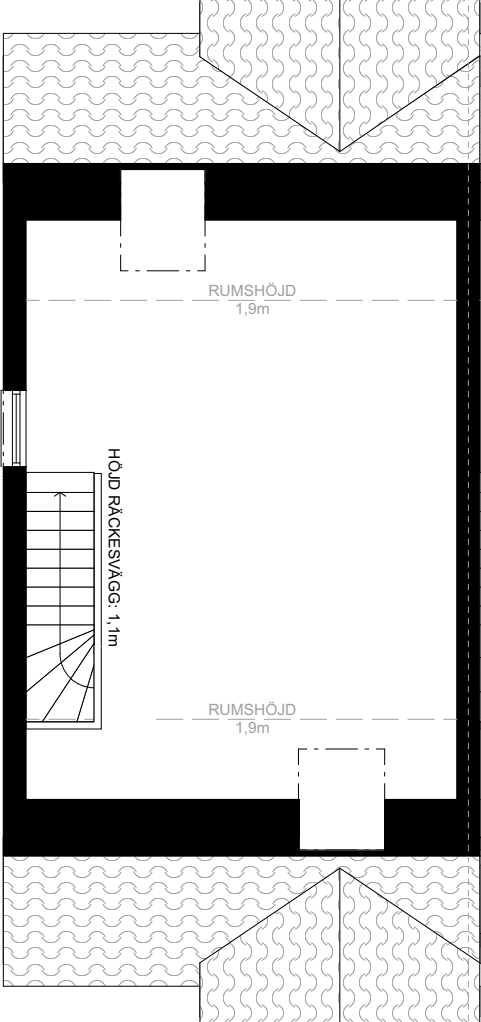
Vindsplan
