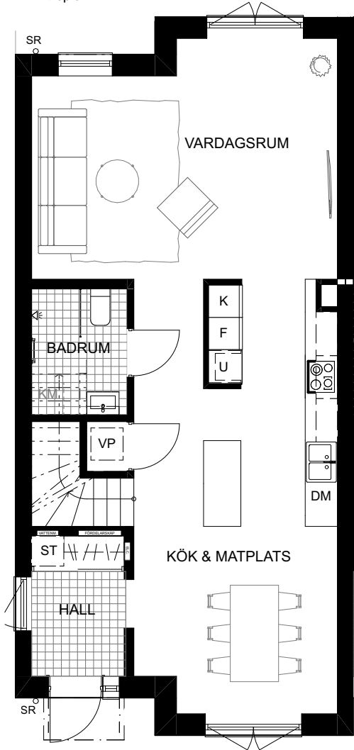
Entréplan
