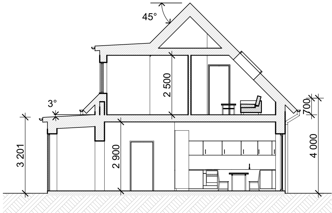
Sektion A-A 1:100
