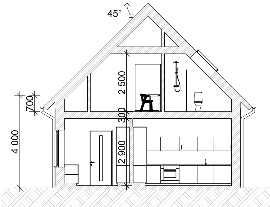
Sektion C-C 1:100
