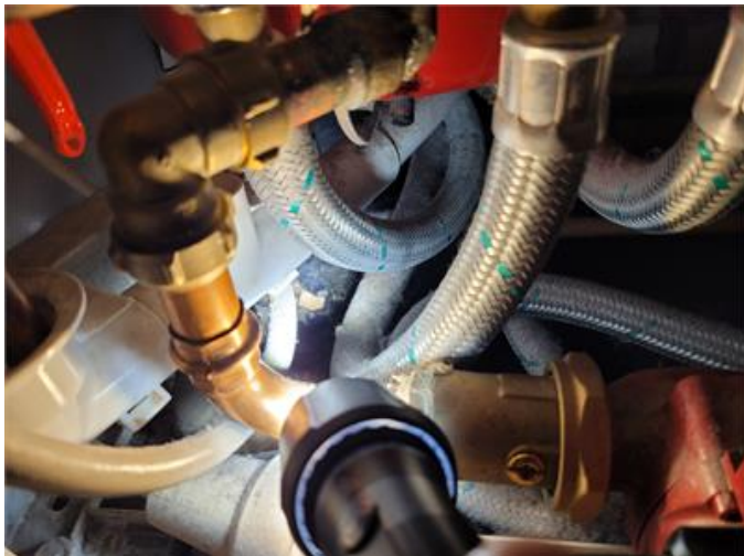
Otättheter på våtrums matta under värmepump.
