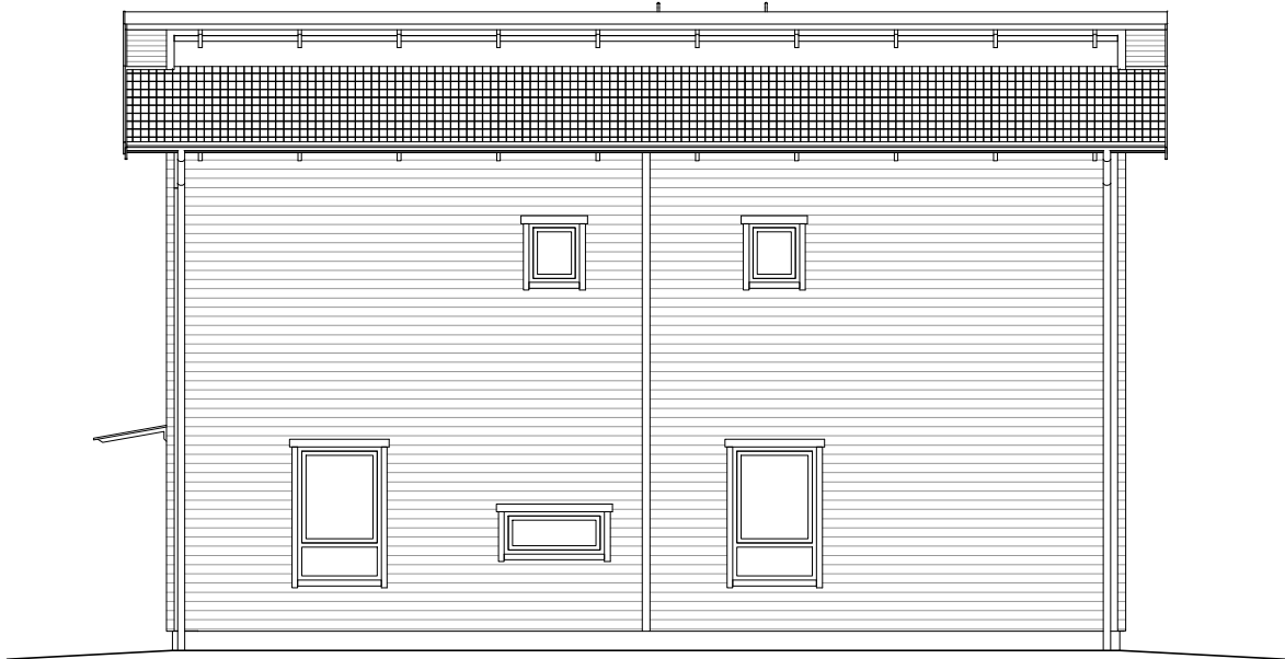
FASAD MOT SYDÖST 1:100 (A1)
