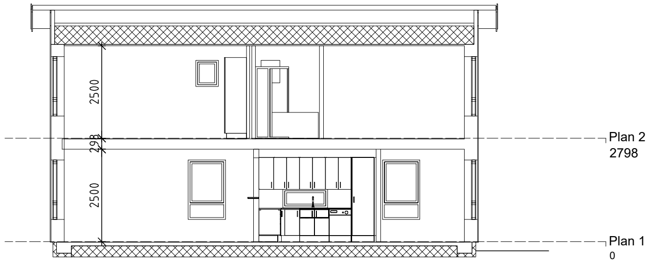
SEKTION 2-2 1:100 (A1)
