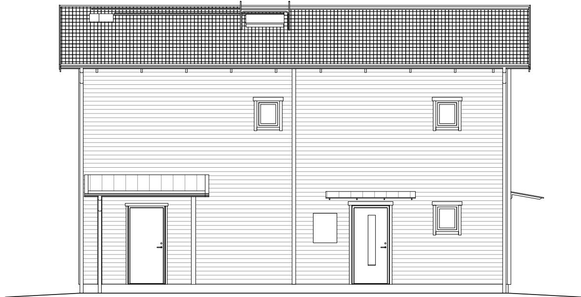
FASAD MOT NORDVÄST 1:100 (A1)
