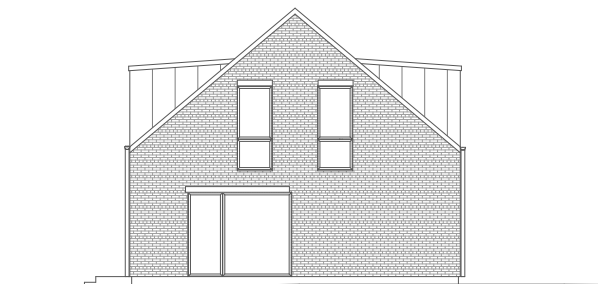
HÖGER GAVEL
