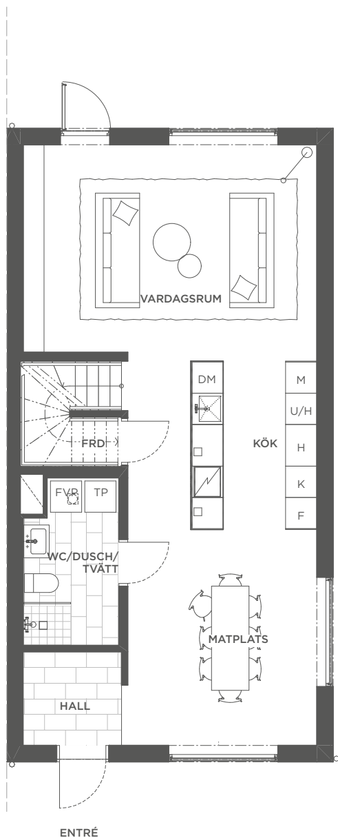
ENTRÉPLAN
