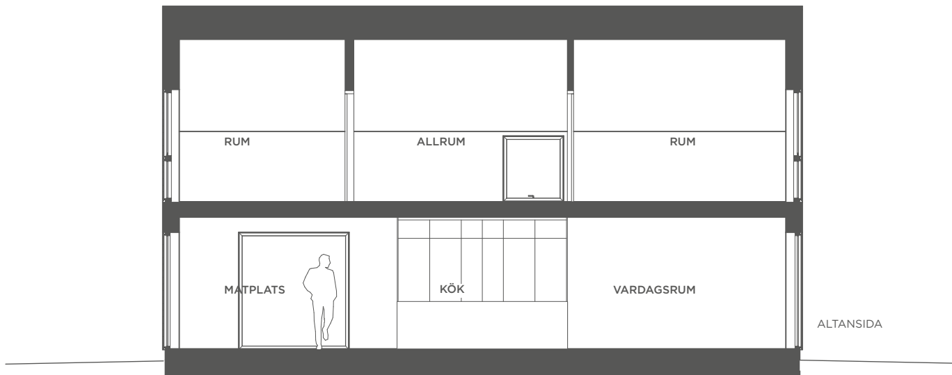
LÄNGDSEKTION CM10
