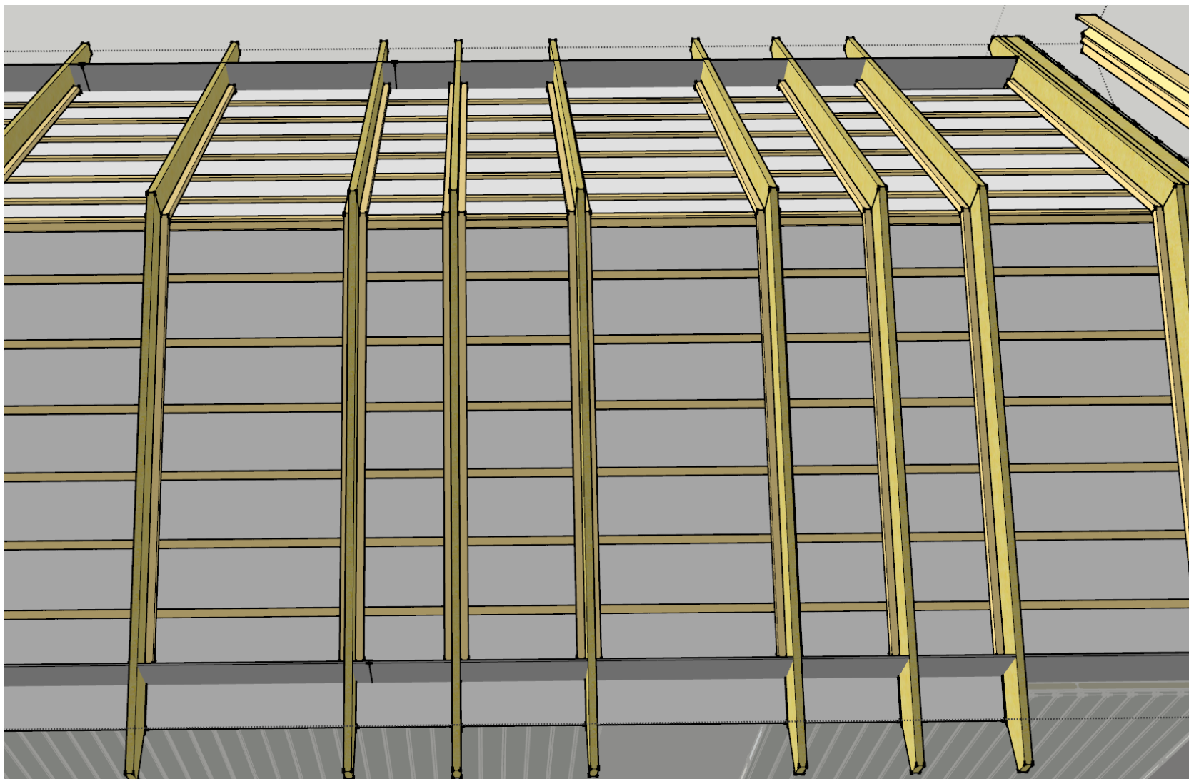
Takstolar över garaget. Innertaket sitter i läkt. För att infästningen mot takstolarna skulle bli stark spikades 45*45 regler längs takstolarna. Vid takfoten monterades utegips (Climaboard).
