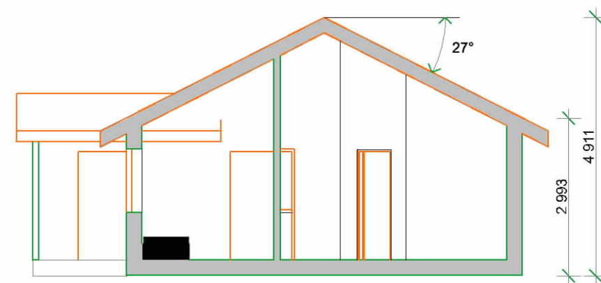
Sektion A 1:100
