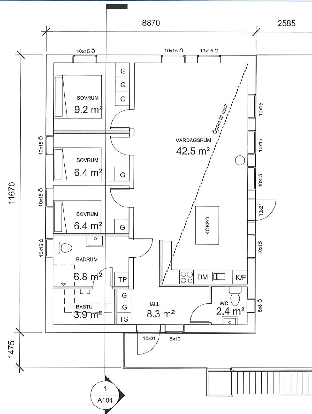
2 - Bottenplan 1 : 100
