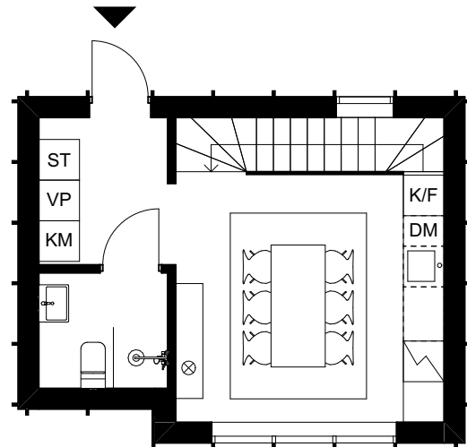
Entréplan
