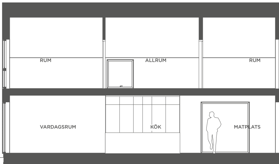
LÄNGDSEKTION CM10
