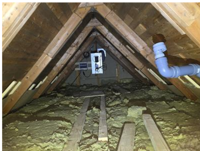
Nockvind: Mikrobiell påväxt i underlagstak. Fläkt nyligen installerad. Vakuumentil till avloppsluftare i utrymmet.
