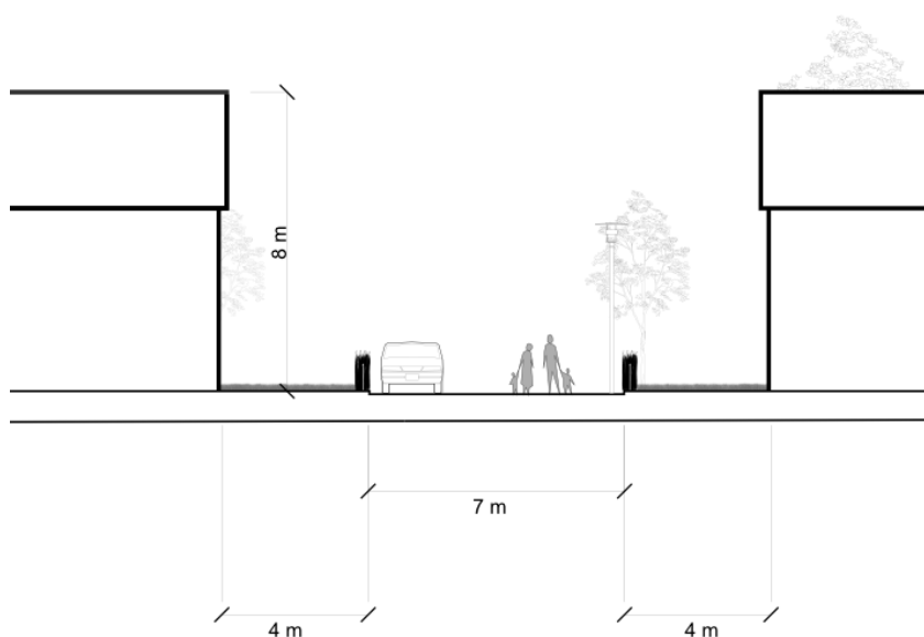
2. Typsektion lokalgata
