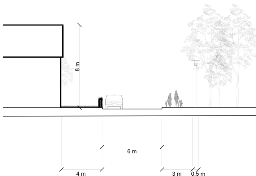
1. Typsektion huvudgata
