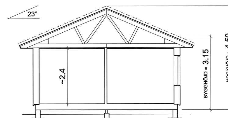
SEKTION A-A.
