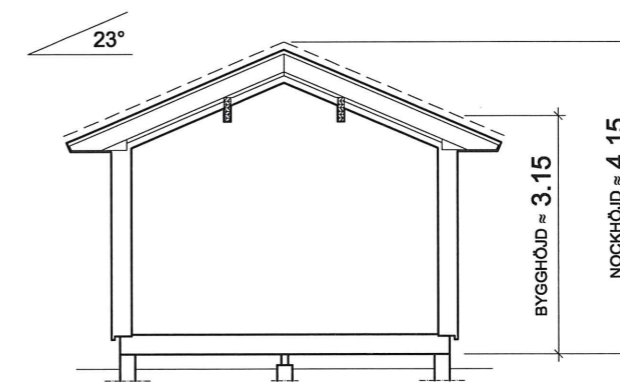
SEKTION B.
