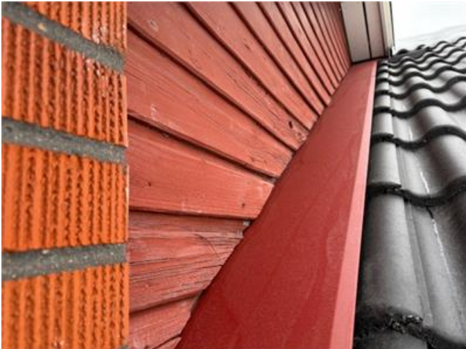
Bilden visar del av fasad där torrsprickor/rötskador förekommer.
