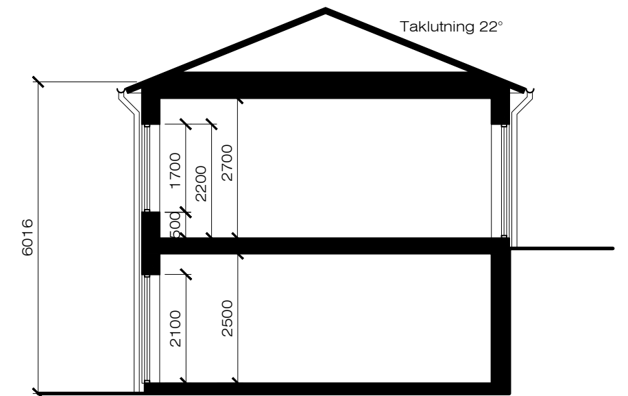
Principsektion
